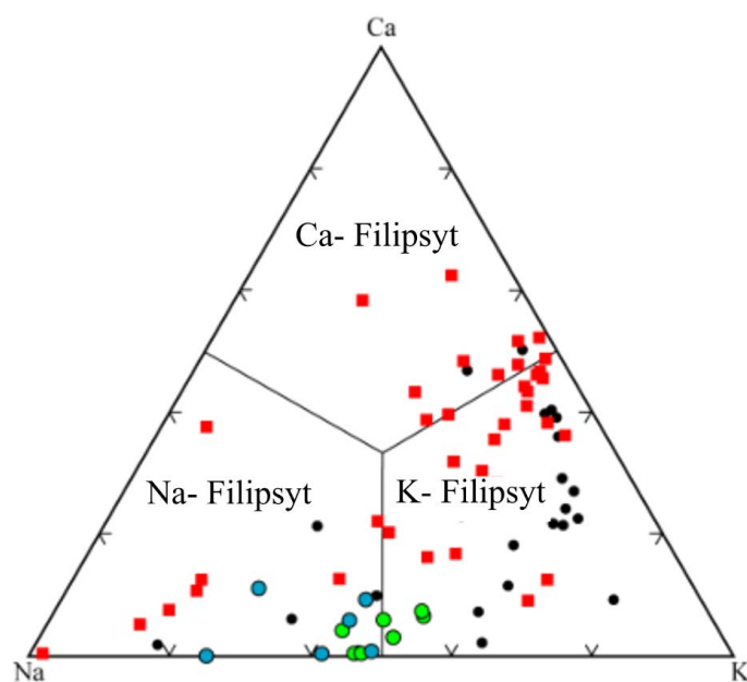
Rys. 1. Diagramm des Zusammensetzungsraums von Phillipsit mit Berücksichtigung der Herkunft einzelner Proben. Die Symbole zeigen die Vorkommen des Phillipsits: rote Quadrate – leere Räume in Basalten, schwarze Kreise – potasose pyroklastische Gesteine, blaue Kreise – alkalische Seesedimente, grüne Kreise – Tiefseesedimente ( www.iza-online.org )
