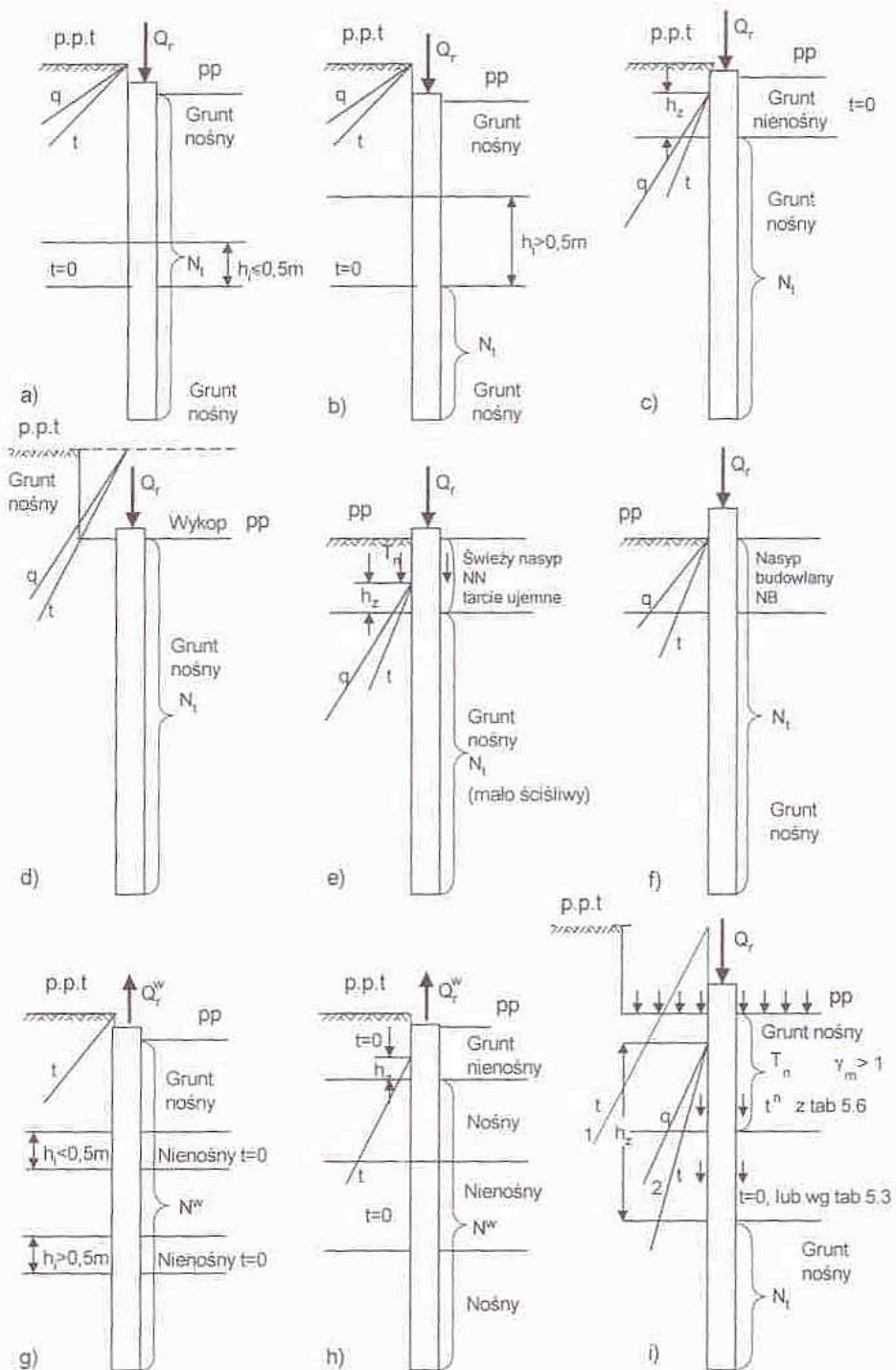
Rys. 5.3. Zasady przyjmowania poziomu odniesienia dla podłoża przewarstwionego gruntami nienośnymi.
