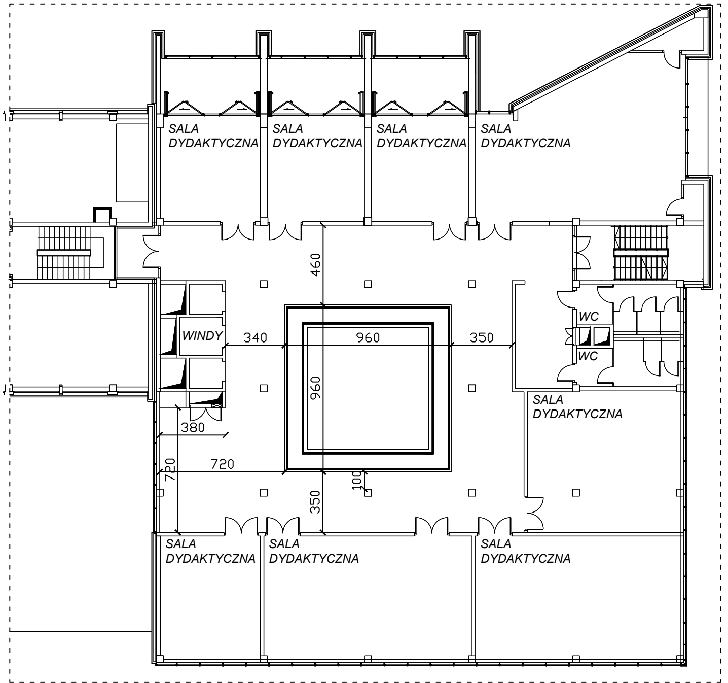
RZUT II PIĘTRA
